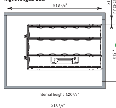
Right hinged door
