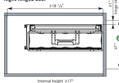
Right hinged door
